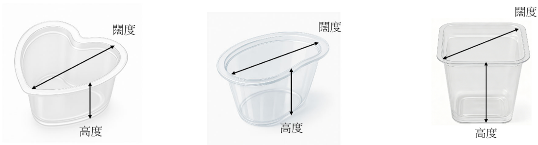
圖 4：展示如何量度非圓口迷你杯的示意圖。
